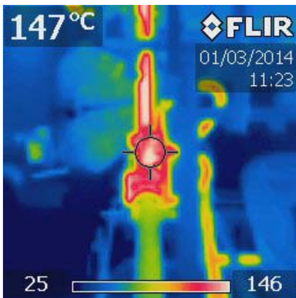
Bare Pipe Temp: 147 C
